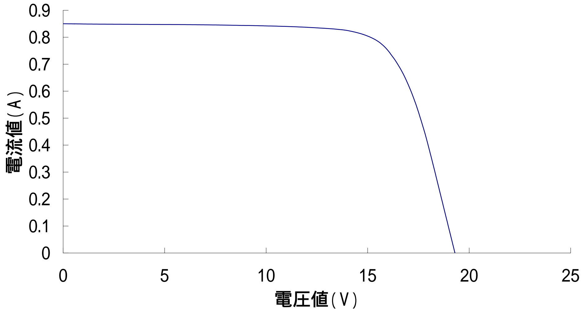
BT 4 3 2 - MRN出力特性図 @1000W/m 2 AM1.5 25
